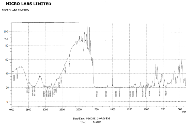
Figure 9: FT-IR spectrum of API-1 + API-2 + Disodium edetate.
